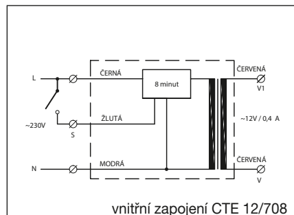
vnitřní zapojení CTE 12/708
